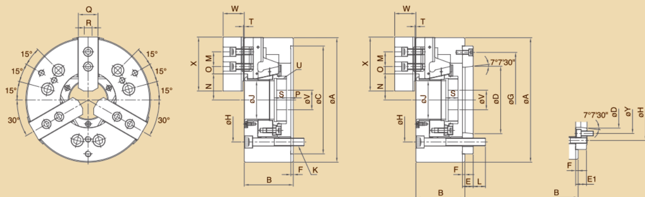
尺寸圖 » Dimensions
